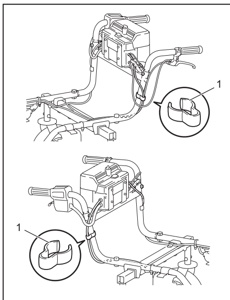
► 1. Clamp
