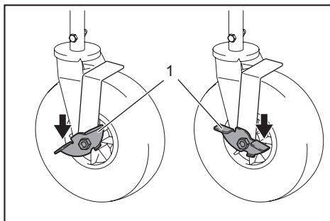
► 1. Pédale
